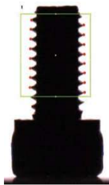
牙距量測
