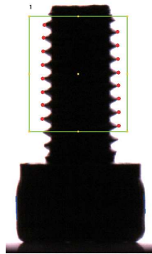
牙距量測
