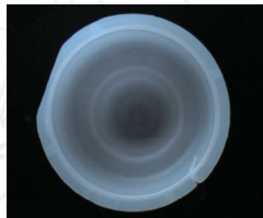
底部裂痕
